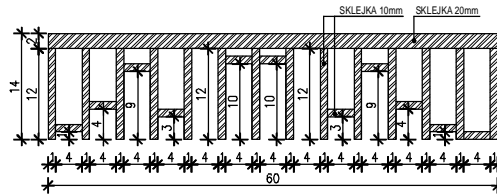
PRZEKRÓJ POZIOMY
