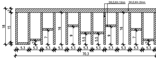
PRZEKRÓJ POZIOMY
